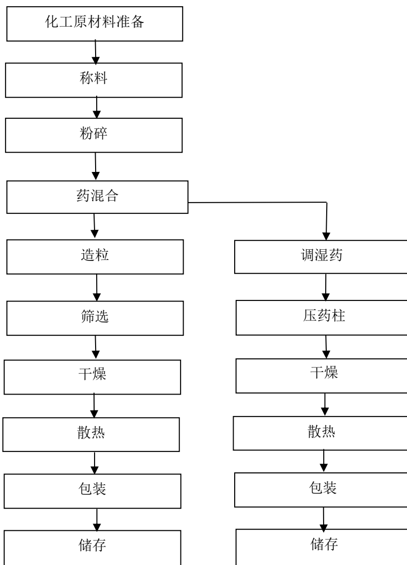
图 2.4-1 亮珠、药柱生产工艺流程图
