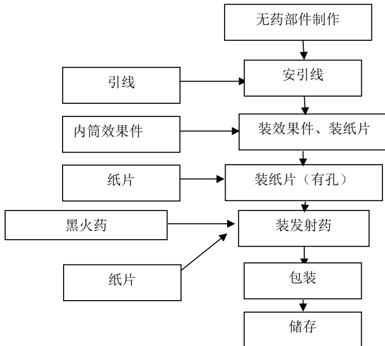
图 2.4-3 组合烟花类产品生产工艺流程图
