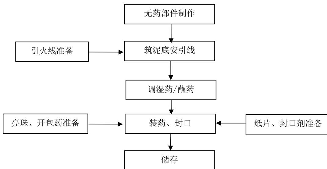
图 2.4-2 效果内筒生产工艺流程图
