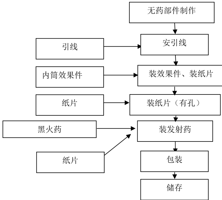
图 2.6-4 礼花类（圆柱型小礼花）生产工艺流程图
