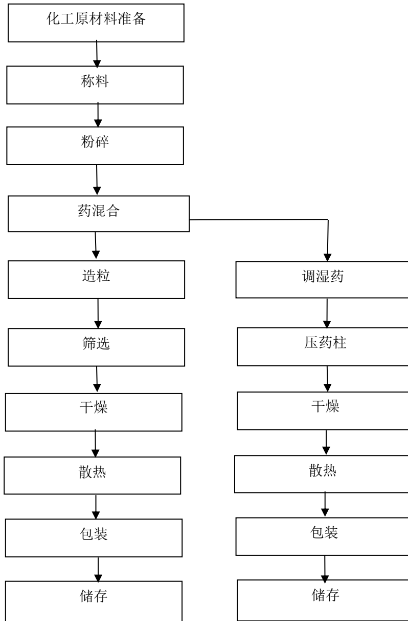
图 2.6-1 亮珠、药柱生产工艺流程图
