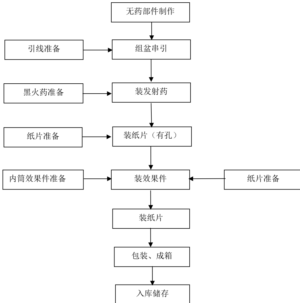
图 2.6-3 组合烟花类产品生产工艺流程图
