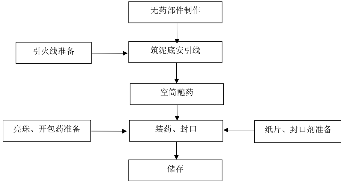
图 2.6-2 效果内筒生产工艺流程图
