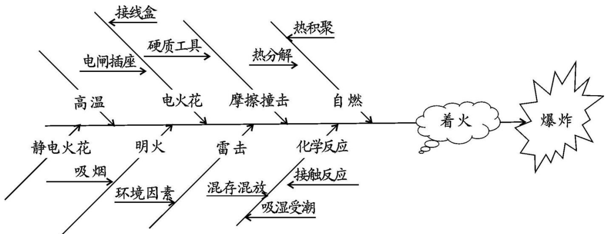
图 3-1 烟花爆竹引爆的因果分析图
