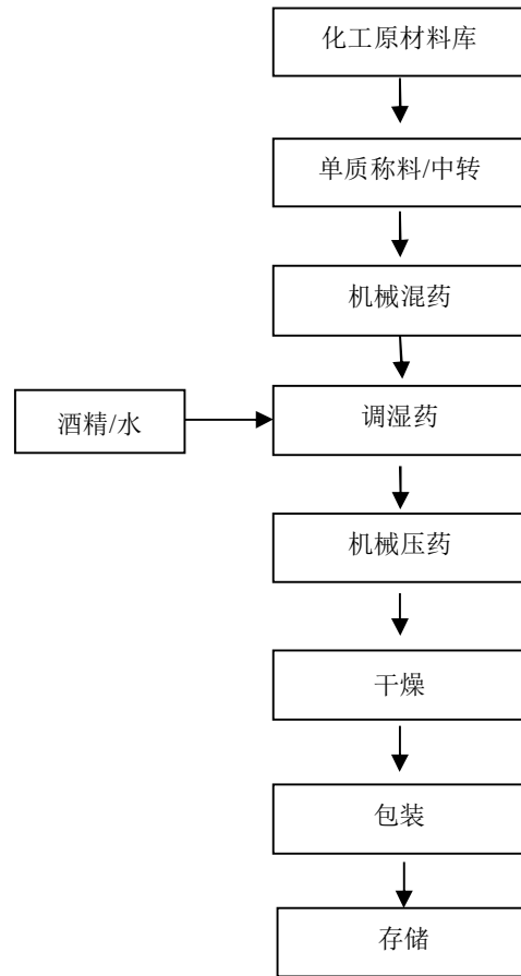
图 2-3：药柱生产工艺流程图
