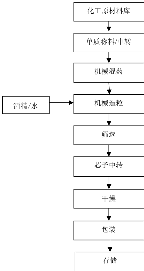
图 2-2：亮珠生产工艺流程图
