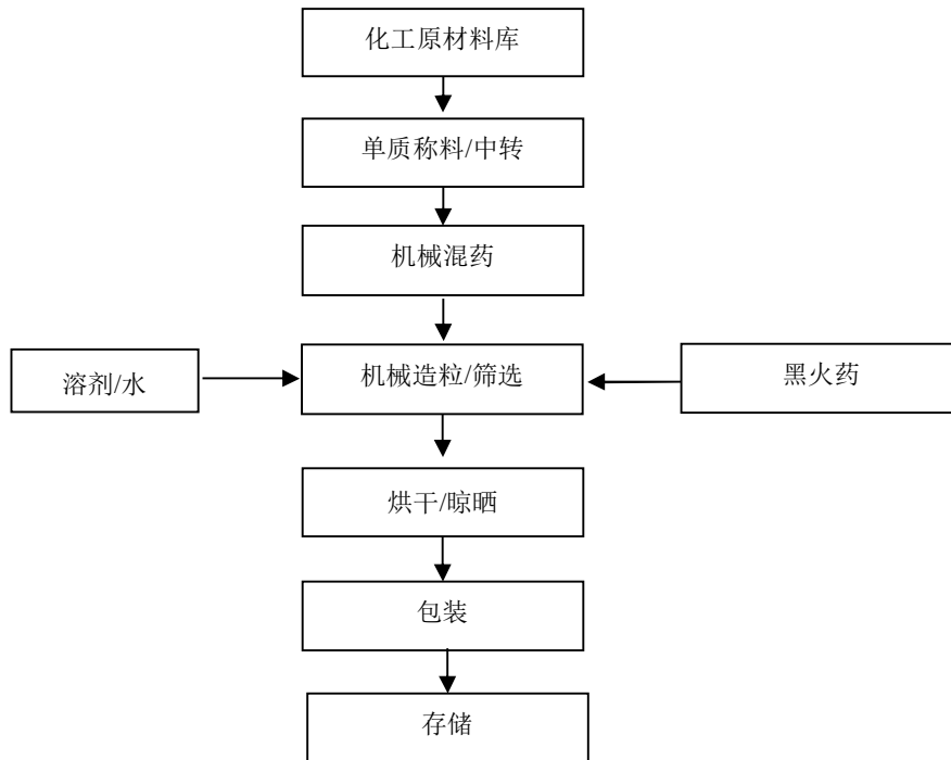
图 2-2：亮珠生产工艺流程图
