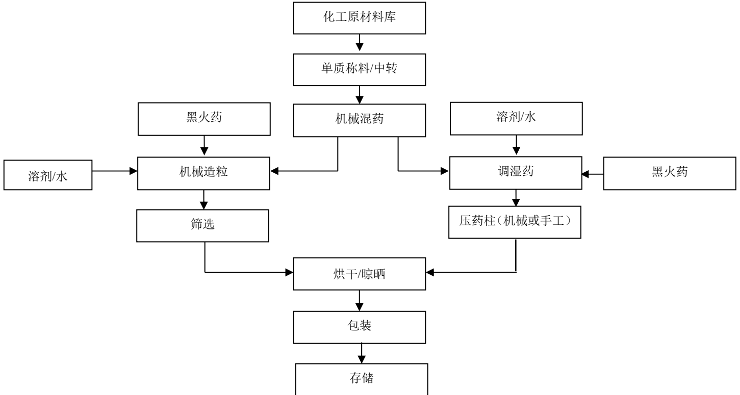
图 2-3：亮珠/药柱生产工艺流程图
