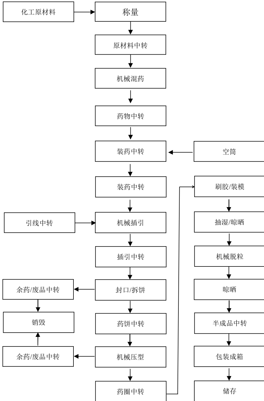
图 2-1：旋转类（彩菊）生产工艺流程图
