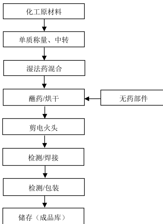
图2.3-3 电点火头生产工艺流程图
