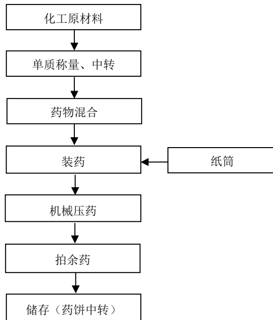
图 2.3-5 笛音效果件生产工艺流程图
