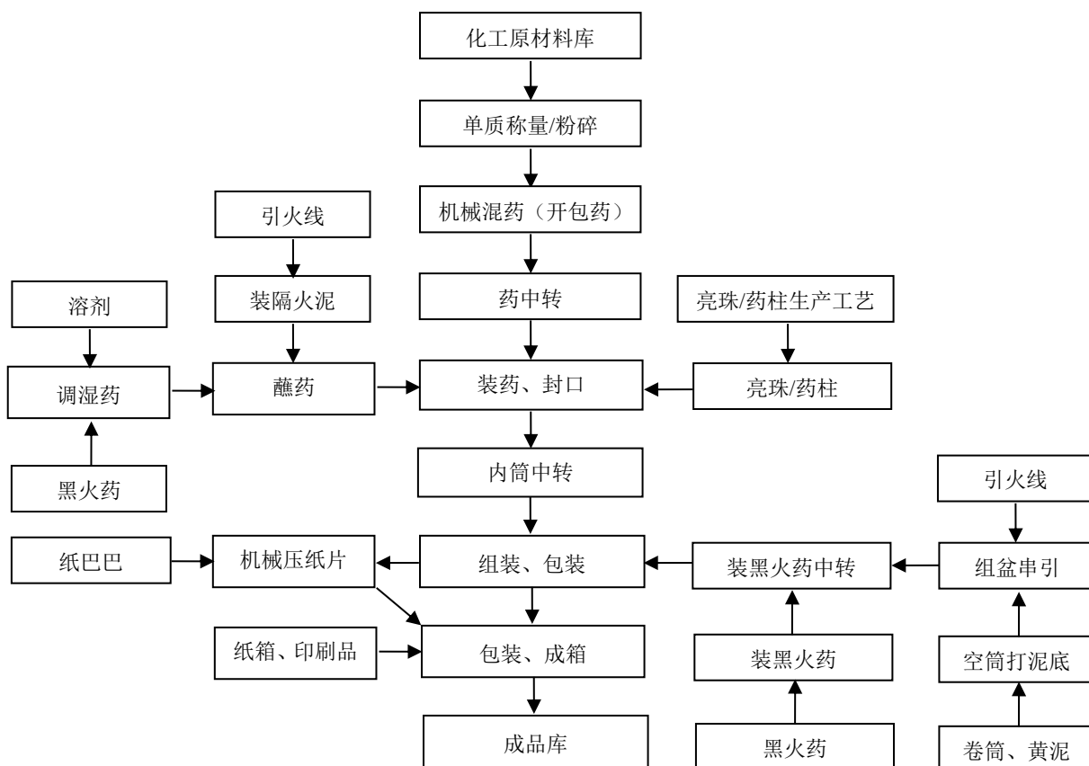
图2.3-1 C、D级组合烟花类生产工艺流程图
