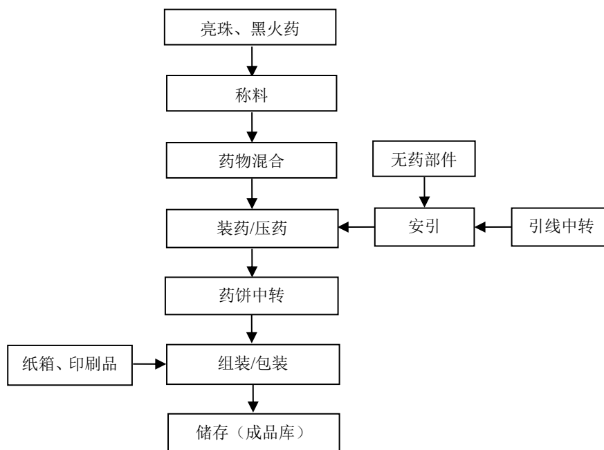
图2.3-2 C级喷花类生产工艺流程图
