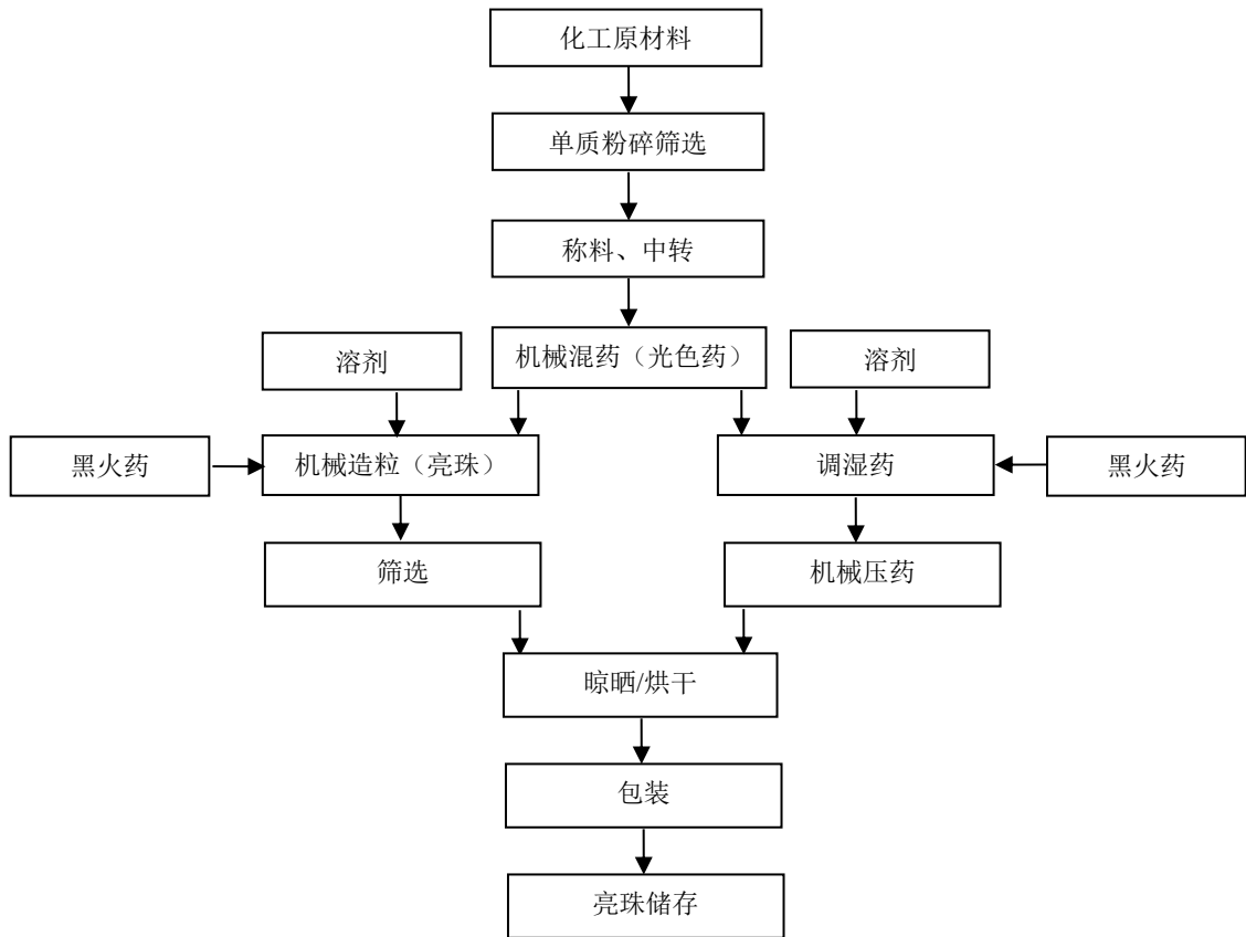
图 2.3-4 烟火药（亮珠/药柱）生产工艺流程图
