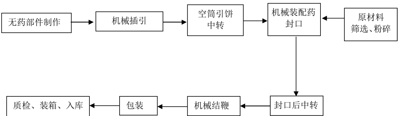
图 2-1：爆竹生产（插引）工艺流程图
