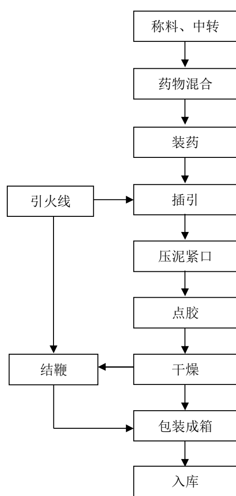
图 2.3-2 爆竹（黑药炮）生产工艺流程图
