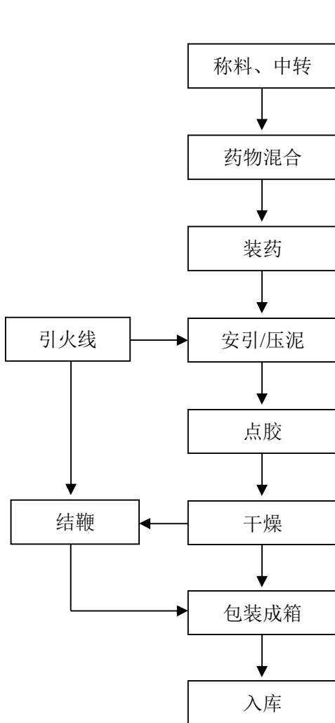
图 2.3-1 爆竹（黑药炮）生产工艺流程图
