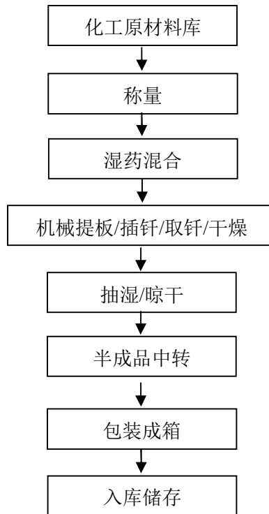
图 2.3-4：玩具类（线香型—电光花）生产工艺流程图
