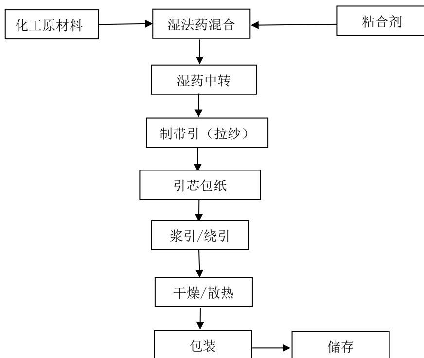
图 2-4-2 带引产品生产工艺流程图
