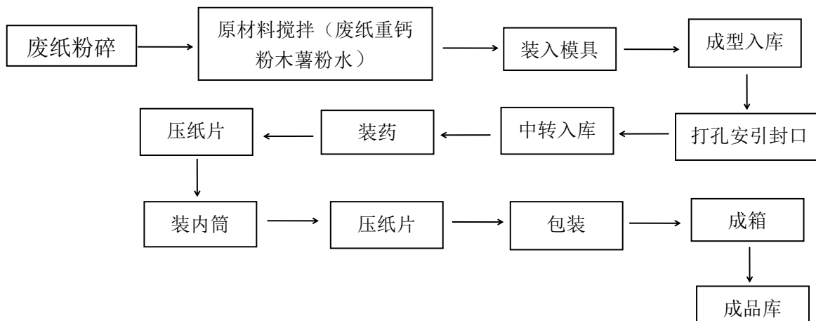
图 2.3-2 组合烟花（模压纸筒）生产工艺流程图
