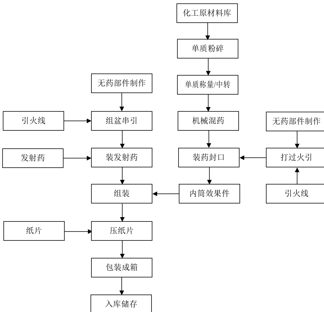
图 2.3-3 组合烟花生产工艺流程图
