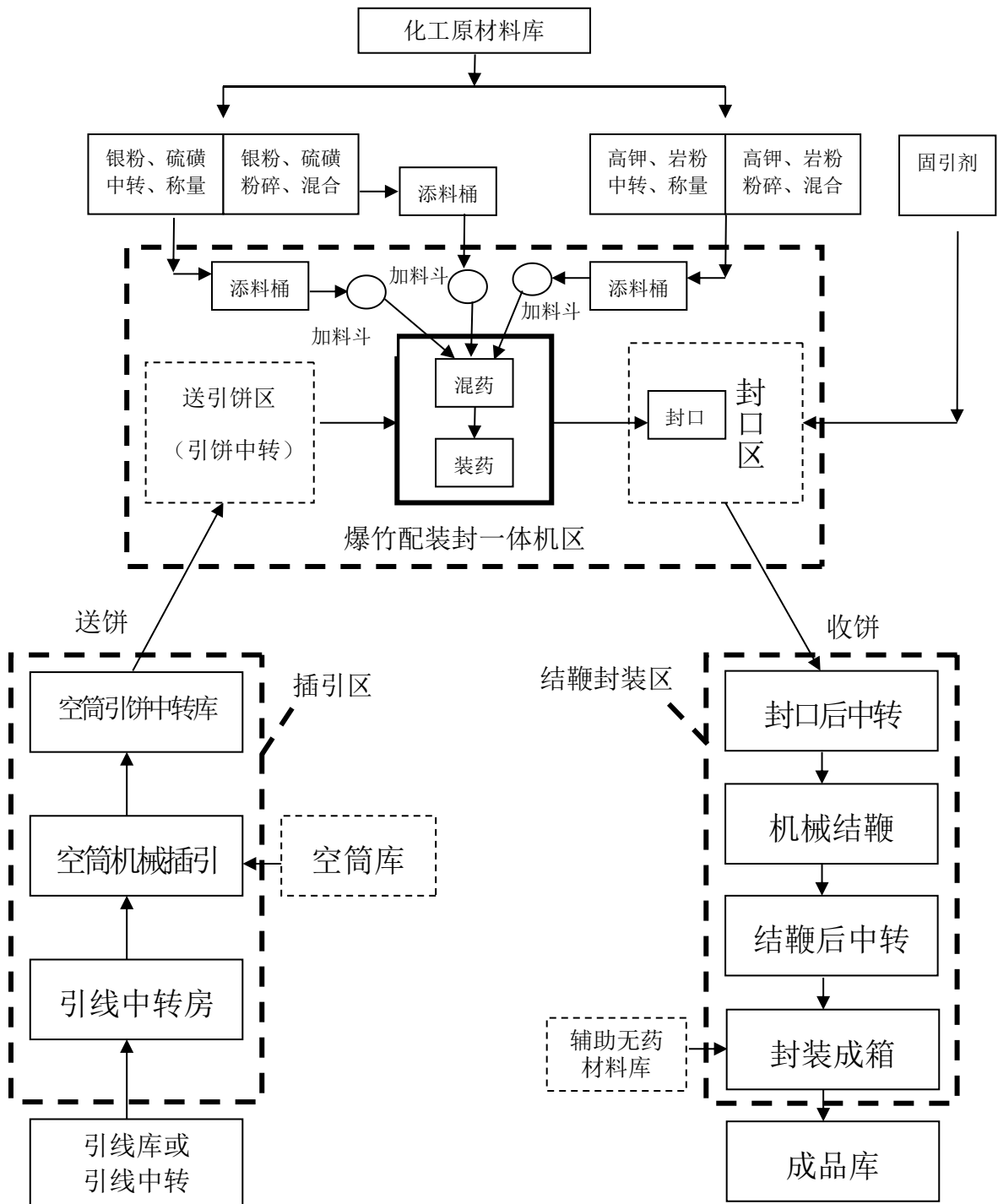
图 2.3-1 爆竹生产无药插引工艺流程图
