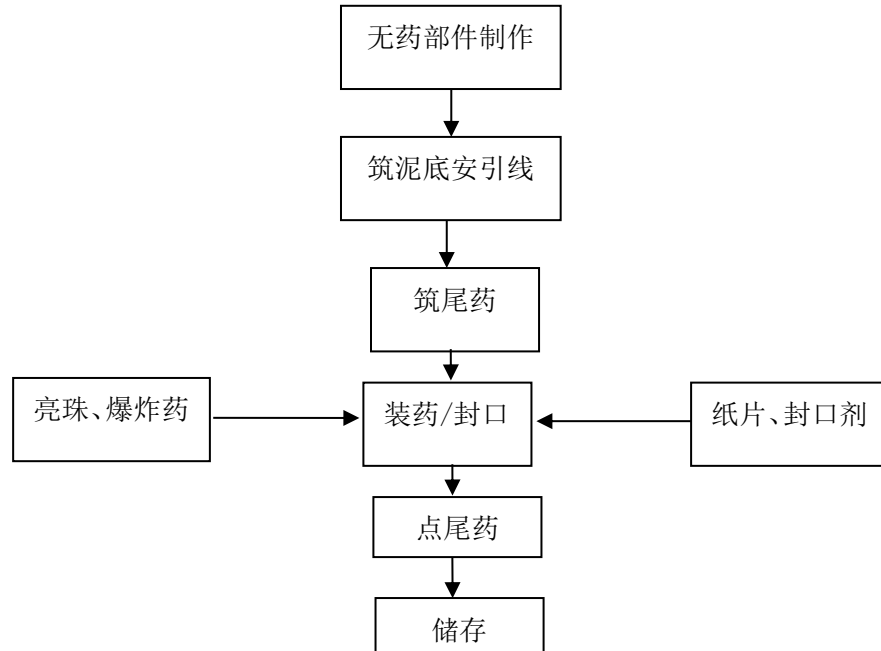
图 2-4-1 效果内筒生产流程图
