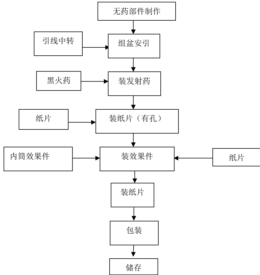
图 2-4-3 组合烟花生产流程图
