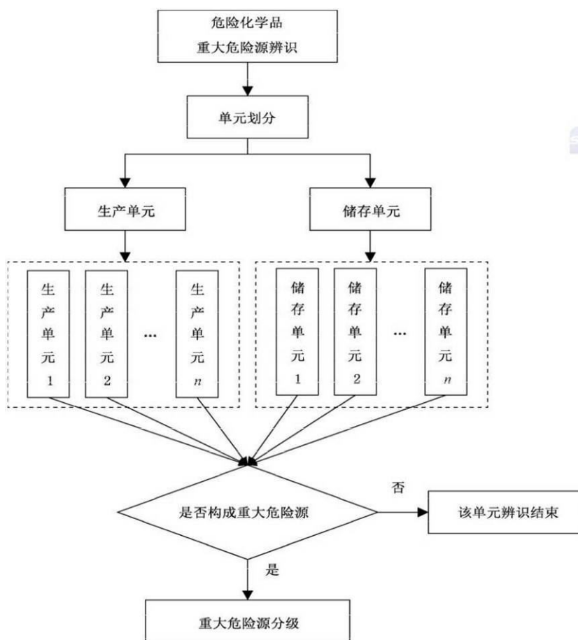
图 3.6-1 重大危险源辨识流程图
