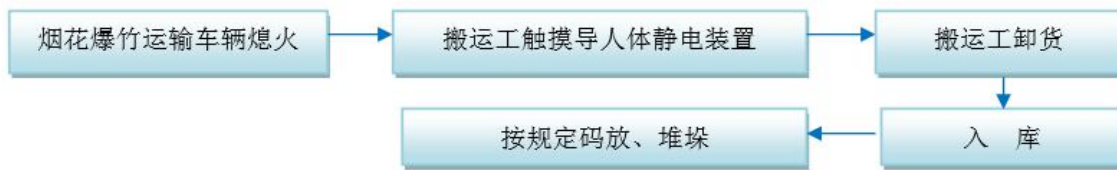
图 2.4-1 入库工艺流程框图
