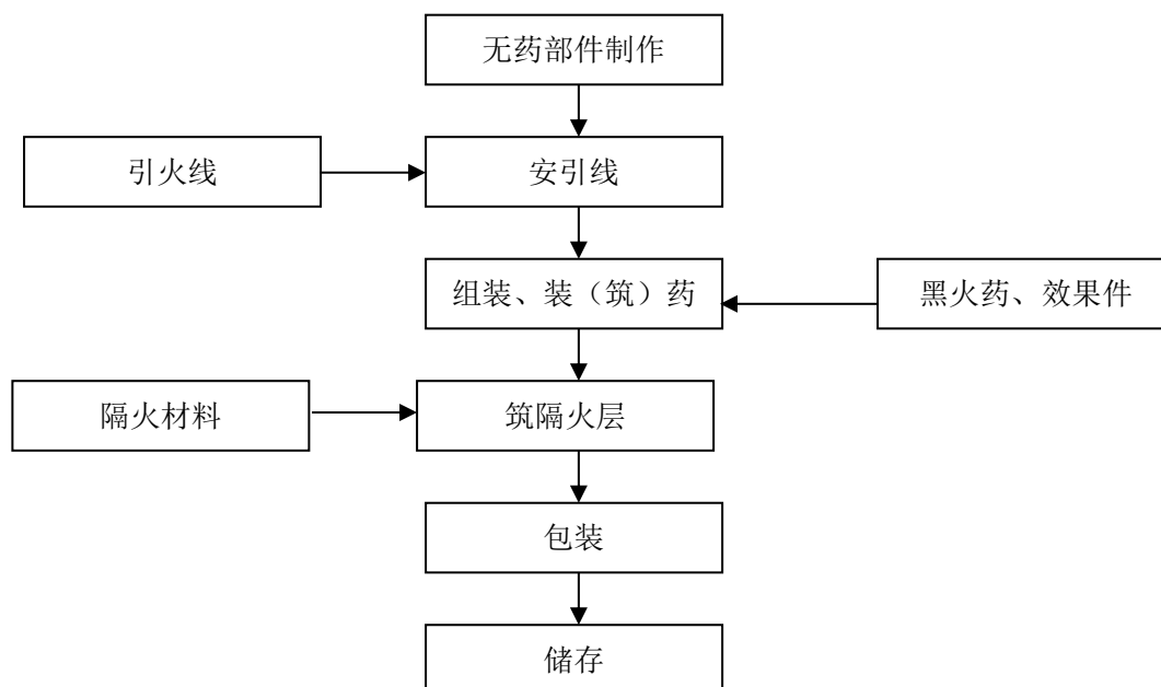
图 2-4-4 吐珠类生产流程图
