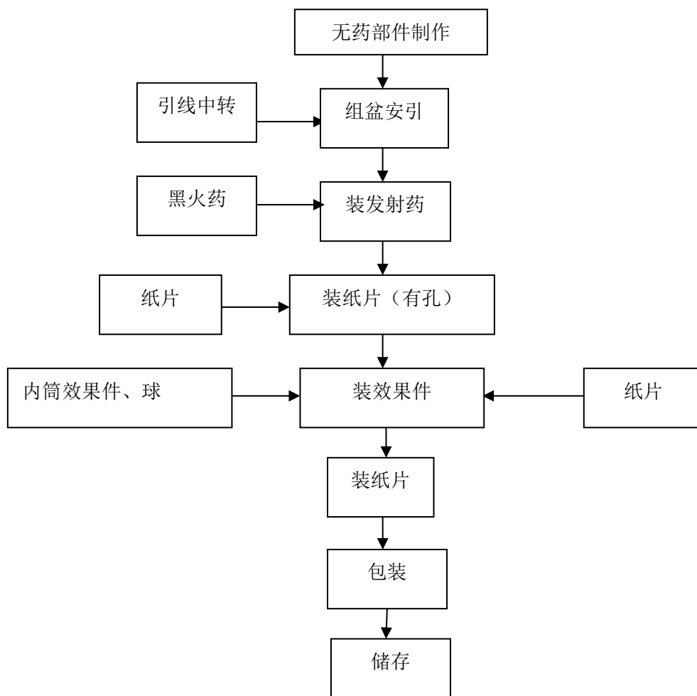
图 2-4-3 组合烟花生产流程图
