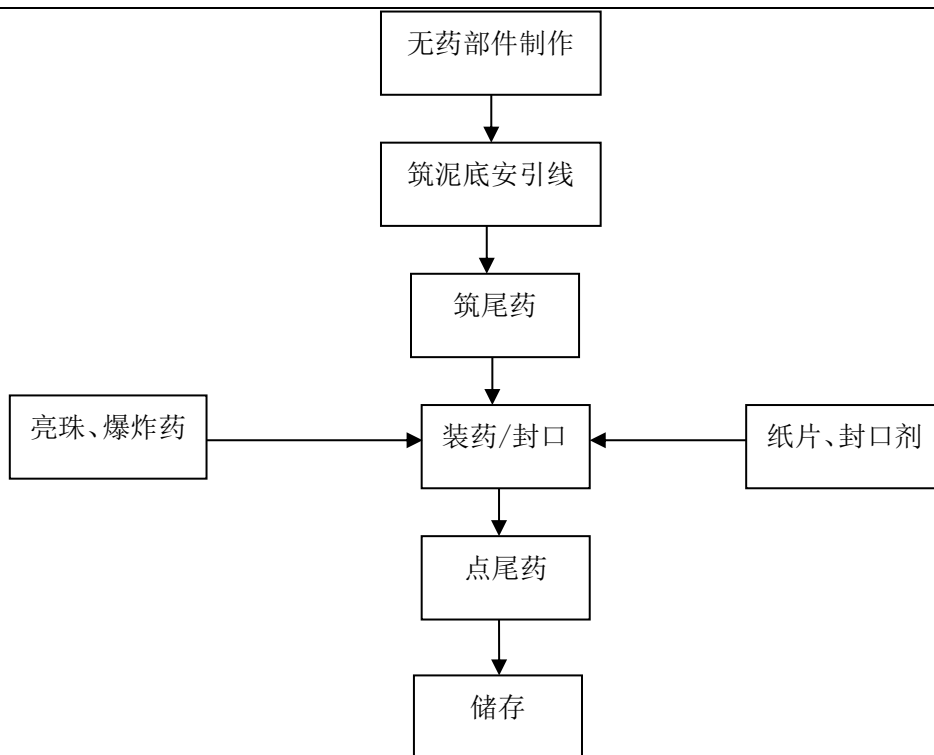
图 2-4-2 效果内筒生产流程
