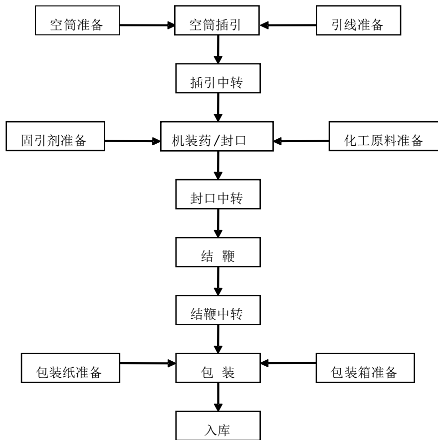
图 2-4-3 爆竹类产品生产工艺流程图
