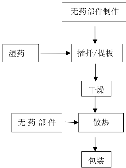
图 2-4-1 玩具类（线香型/电光型）生产工艺流程图
