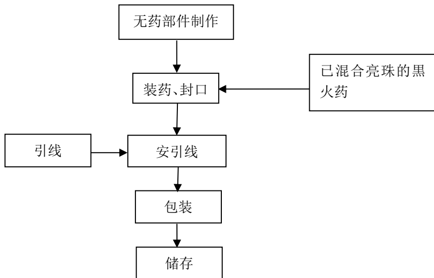
图 2-4-2 喷花类生产工艺流程图
