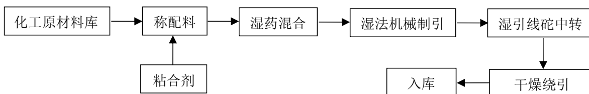
图 2-3：引火线（裁引）生产工艺流程图
