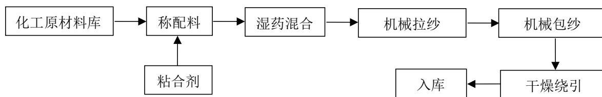
图 2-4：引火线（带引）生产工艺流程图
