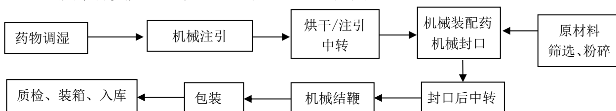
图 2-1：爆竹生产（注引）工艺流程图
